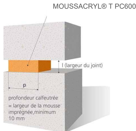
Croquis 3 : Coupe transversale du joint
