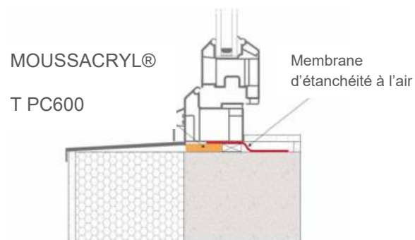
Croquis 15 : Exemple d'étanchéité sous pièce d'appui
