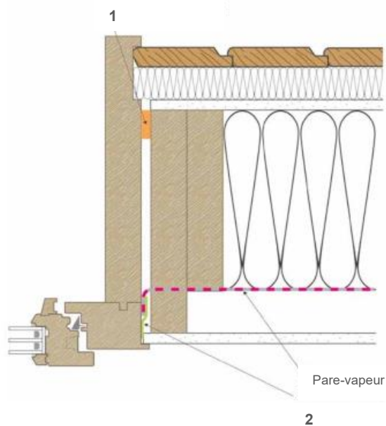
Croquis 25 : Tableau de menuiserie – pose en applique
