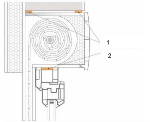
Croquis 27 : Linteau et coffre de volet roulant – pose en tunnel
