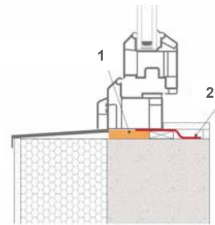
Croquis 28 : Appui de menuiserie – pose en tunnel
