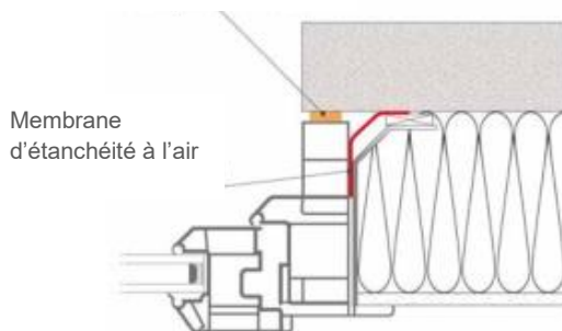
Croquis 13 : Exemples d'étanchéité entre tableau et menuiserie
