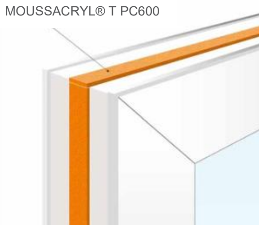
Croquis 8-3 : Raccords d'angle de deux extrémités continues (pose en tunnel)
