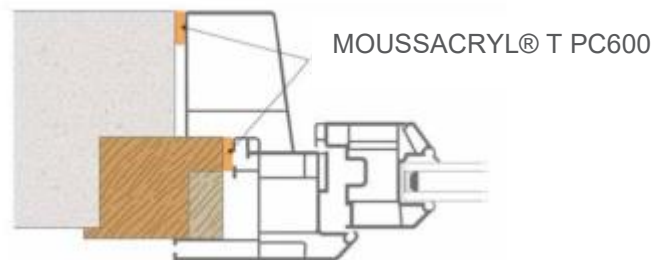
Croquis 17 : Mise en œuvre en rénovation
