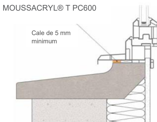
Croquis 11 : Exemples d'étanchéité sous pièce d'appui
