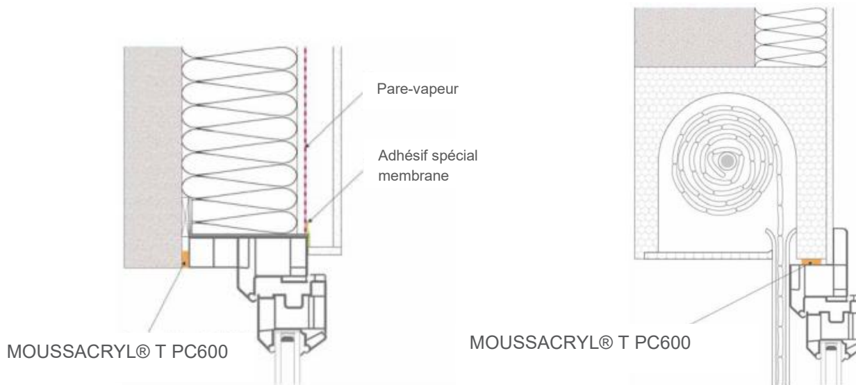
Croquis 12 : Exemples d'étanchéité sous linteau
