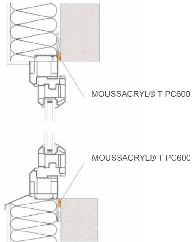
Croquis 16 : Pose en applique extérieure
