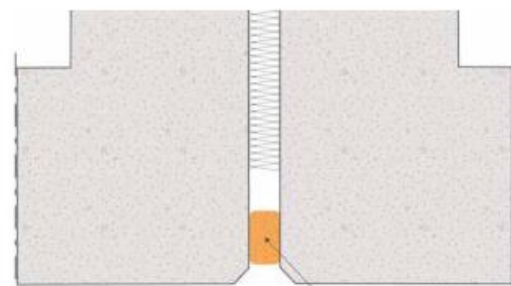
Croquis 21 : Joint entre éléments de béton banché
