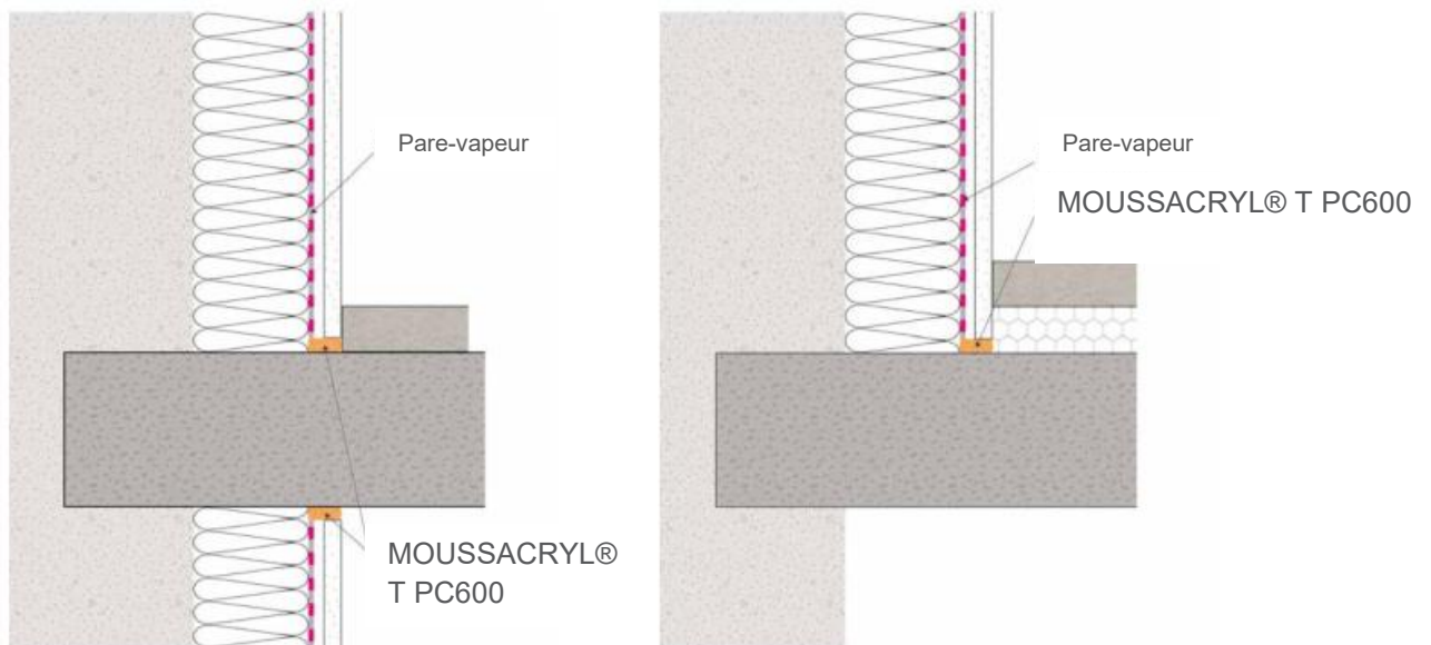
Croquis 32 : Etanchéité du doublage sur mur en maçonnerie
