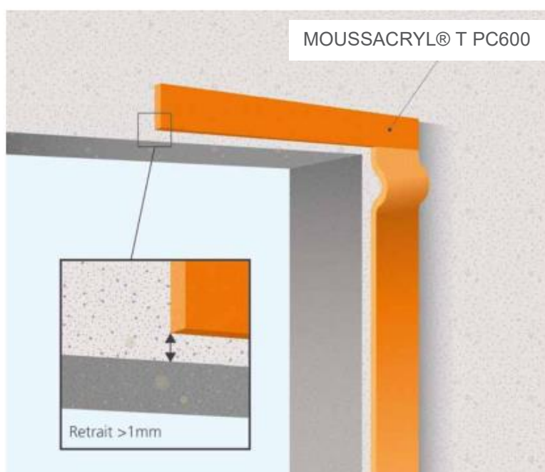
Croquis 8-1 : Raccords d'angle de deux extrémités continues (pose en applique)
