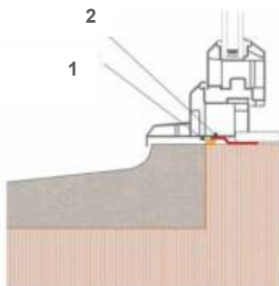
Croquis 29 : Tableau de menuiserie – pose en feuillure
