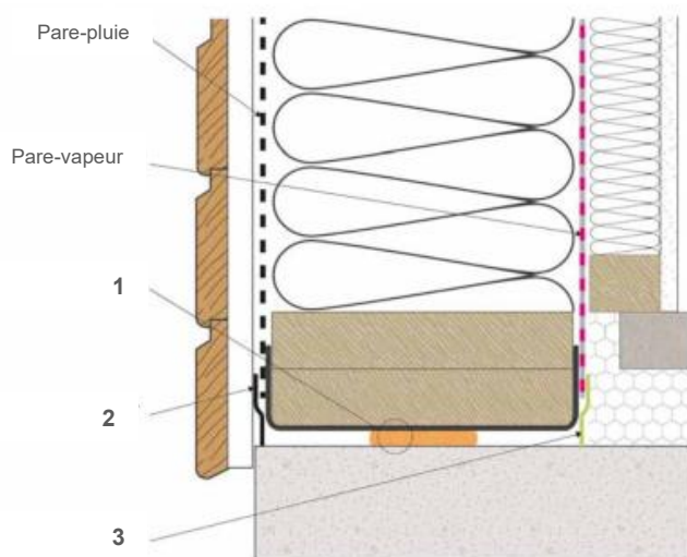
Croquis 26 : Liaison lisse basse et maçonnerie
