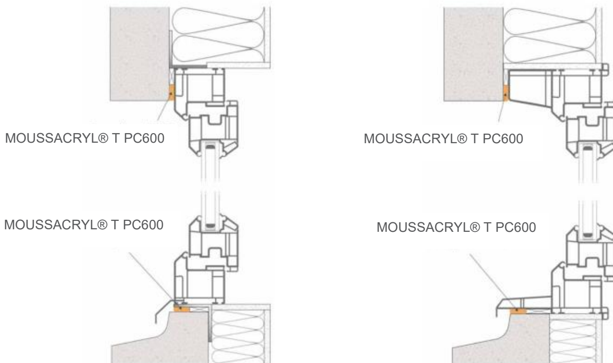
Croquis 9 : Pose en applique intérieure avec appui décalé
