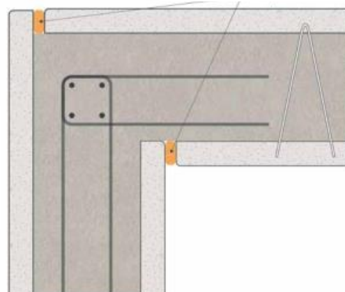
Croquis 22-2 : Joint béton / liaison d'angle
