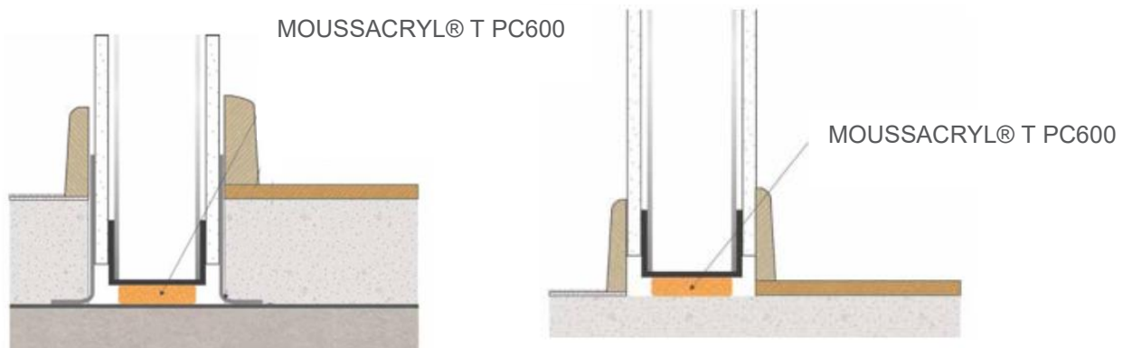
Croquis 31 : Etanchéité sous cloison séparatives
