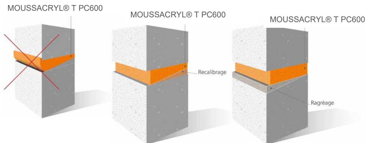
Croquis 5 - Surface de contact
