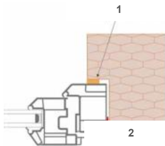
Croquis 29 : Tableau de menuiserie – pose en feuillure
