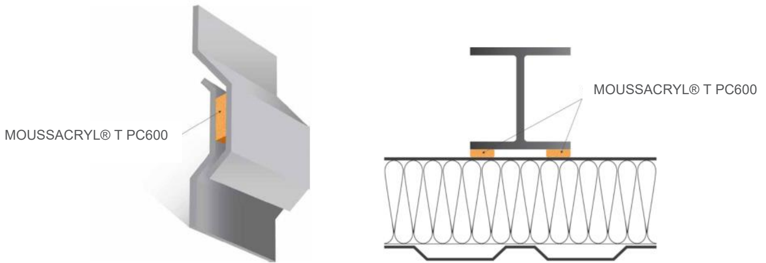
Croquis 33 : Etanchéité en bardage
