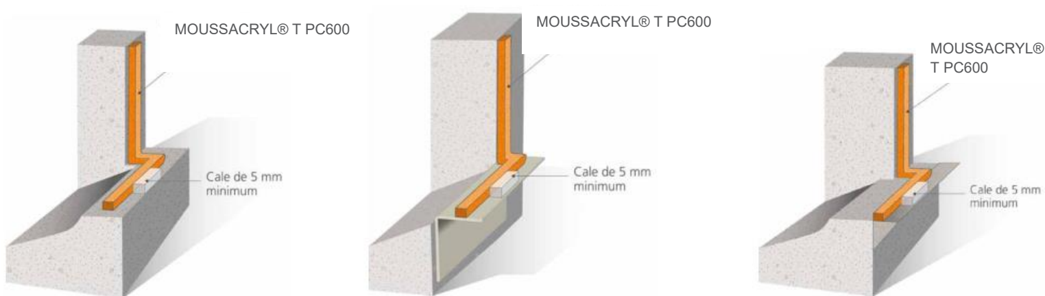
Croquis 10 : Pose sous appui de fenêtre
