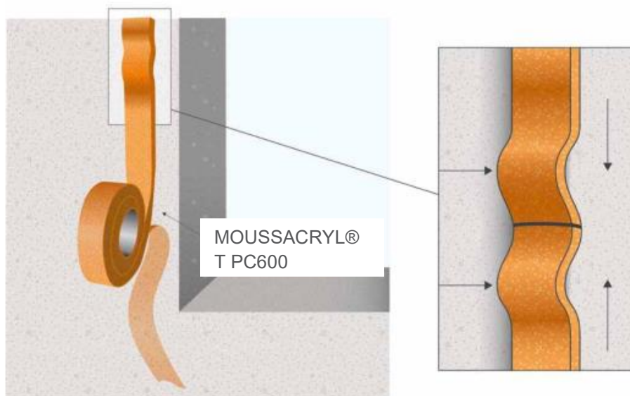
Croquis 7 : Raccords bout à bout de deux extrémités
