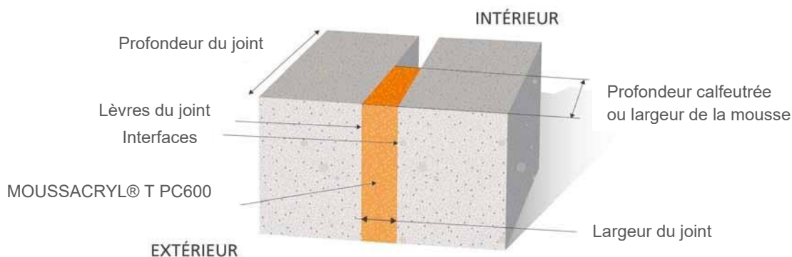
Croquis 1 : Terminologie relative aux joints
