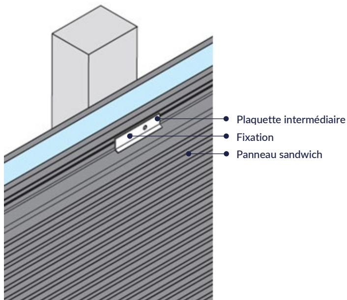
Plaquette de répartition intermédiaire
