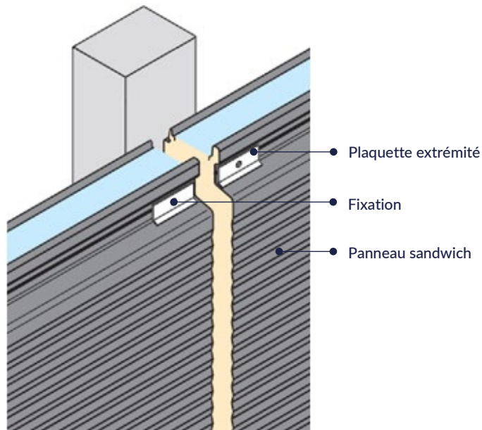
Plaquette de répartition extrémité
