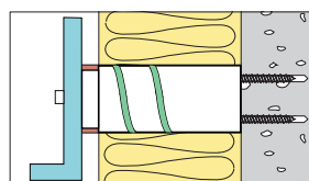
Fixation de la structure
