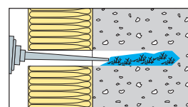
Injection du scellement
