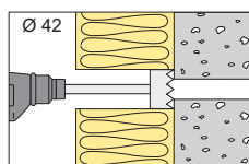
Carottage de l'isolant Ø 42
