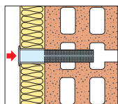
Mise en place du tamis et coupé à la longueur
